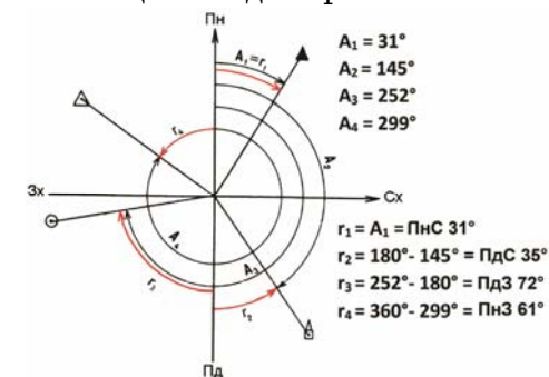
Мал. 47. Співвідношення румбів і азимутів
