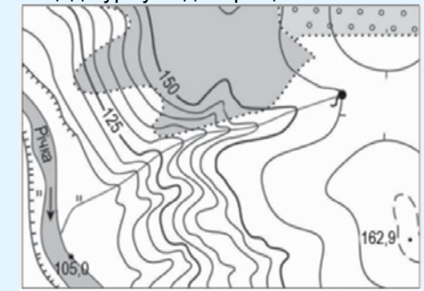
Масштаб 1 : 10 000 Суцільні горизонталі проведено через 5 м
