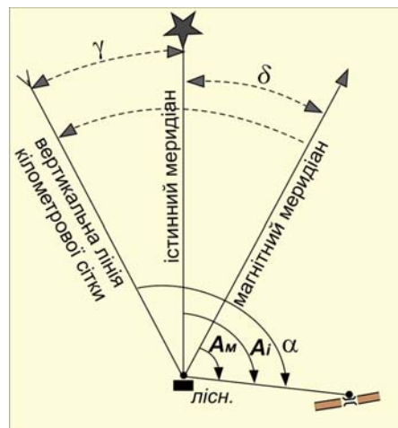
Мал. 46. Кути орієнтування на топографічних картах
