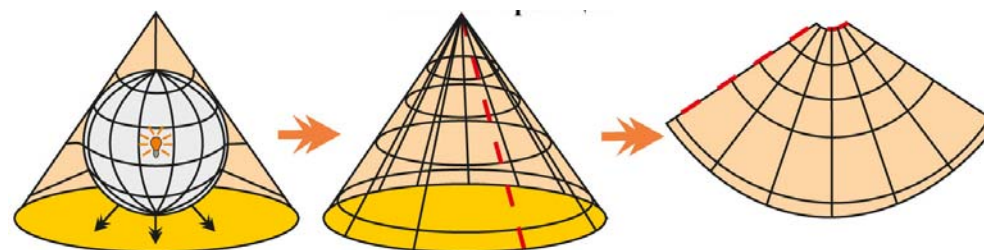
Мал. 31. Створення картографічної сітки у конічній проекції
