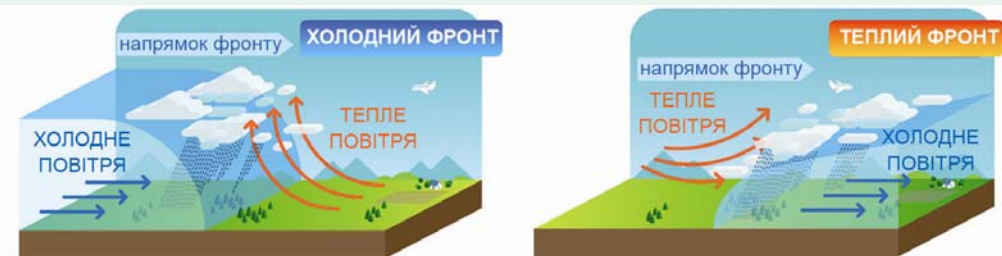
Мал. 99. Атмосферні фронти
