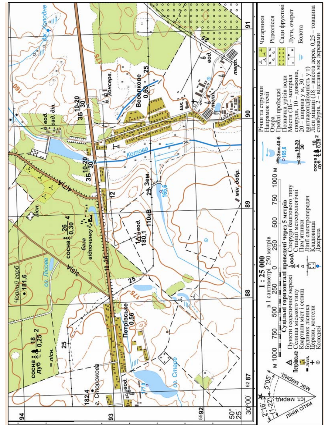
Мал. 36. Фрагмент аркуша топографічної карти
