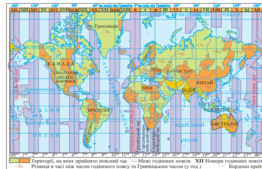
Мал. 10. Картоschema годинних поясів світу
