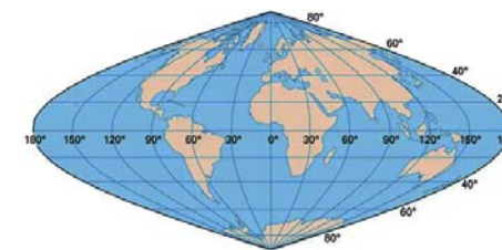
Мал. 32. Одна з умовних проекцій, яку називають псевдоциліндричною
