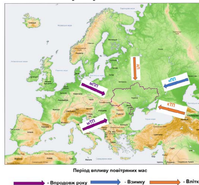
Мал. 97. Циркуляція повітряних мас над територією України
