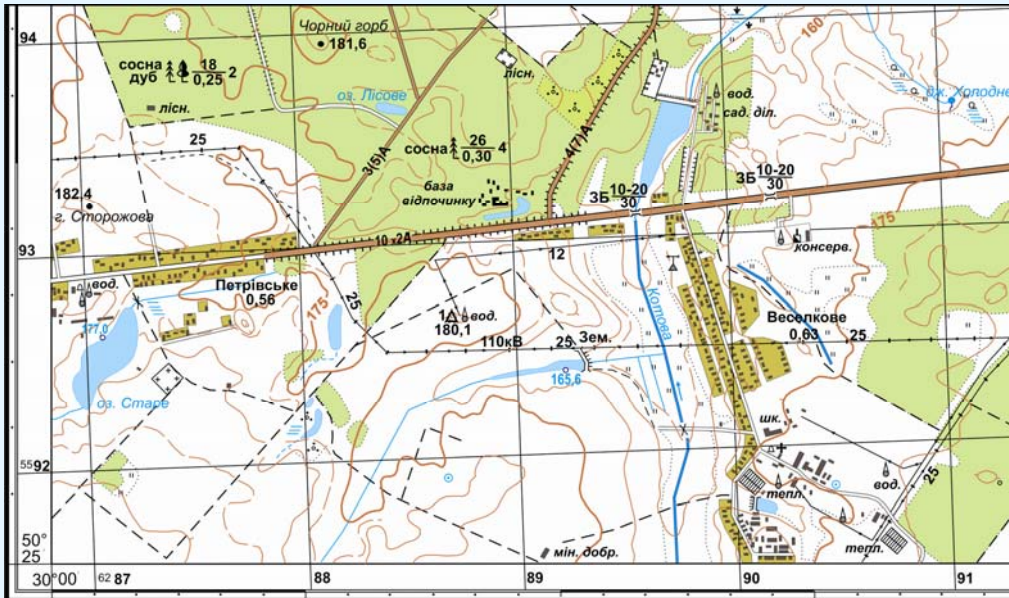
Мал. 45. Фрагмент аркуша топографічної карти М-36-49-В-а
