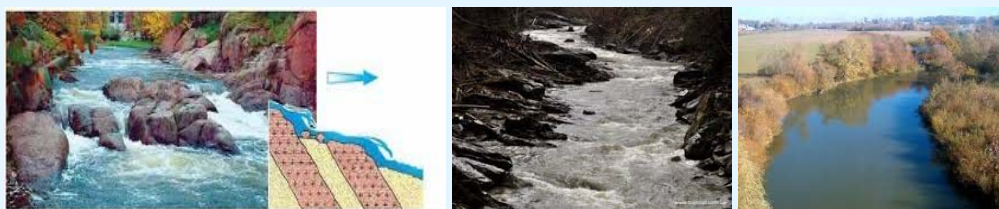
Мал. 129. Річкові долини та їх зв'язок із геологічною будовою та рельєфом
