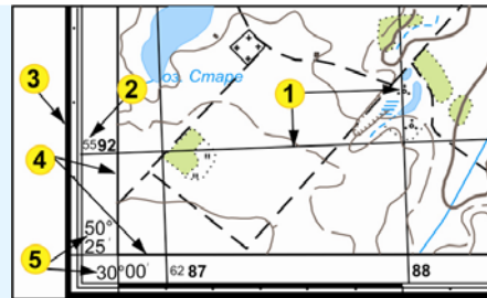
Мал. 40. Елементи топографічної карти
